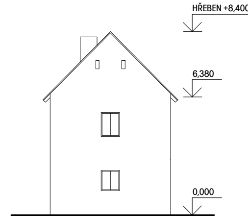
POHLED JIHOVÝCHODNÍ
