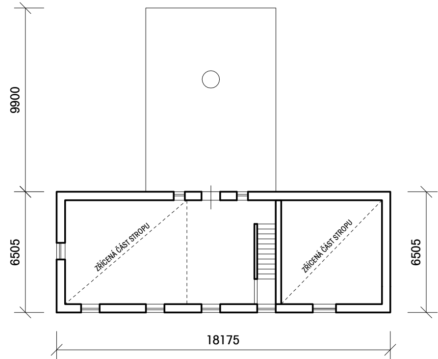
PŮDORYS 2NP
