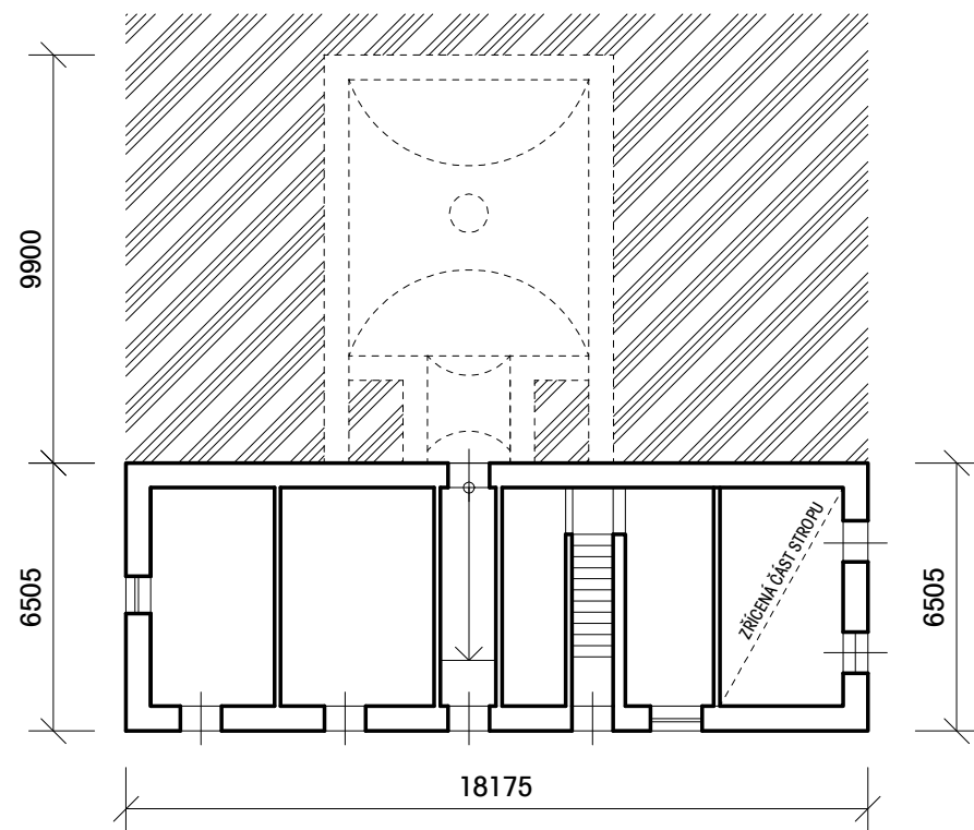
PŮDORYS 1NP
