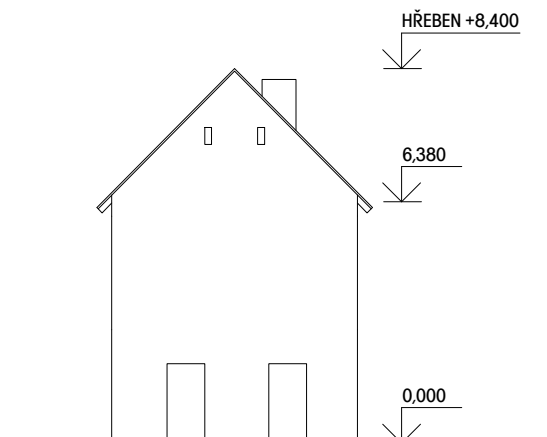
POHLED SEVEROZÁPADNÍ
