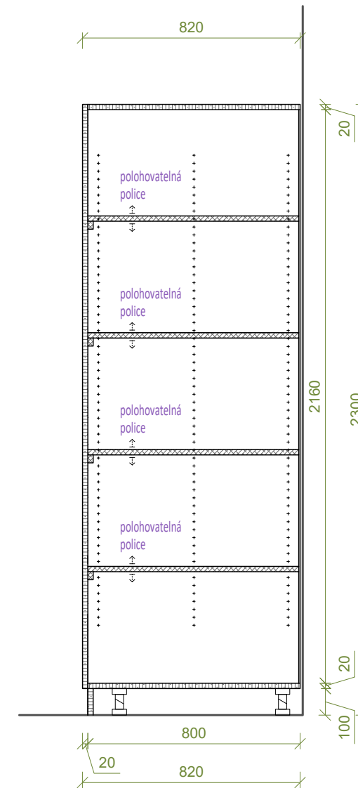
ŘEZ A-A
