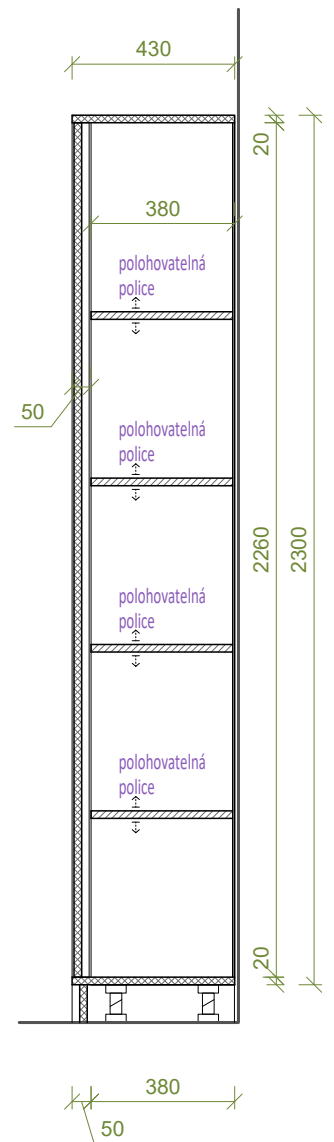
ŘEZ A-A
