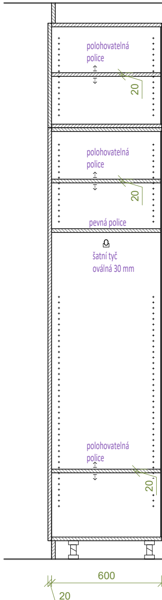
ŘEZ A-A
