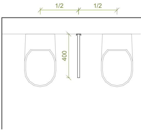
PŮDORYS
