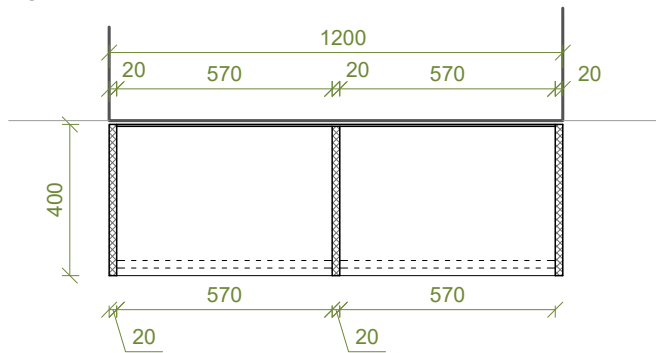
PŮDORYS 2
