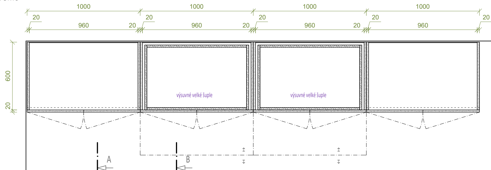
PŮDORYS
