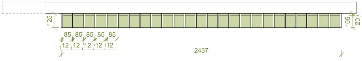
PŮDORYS
