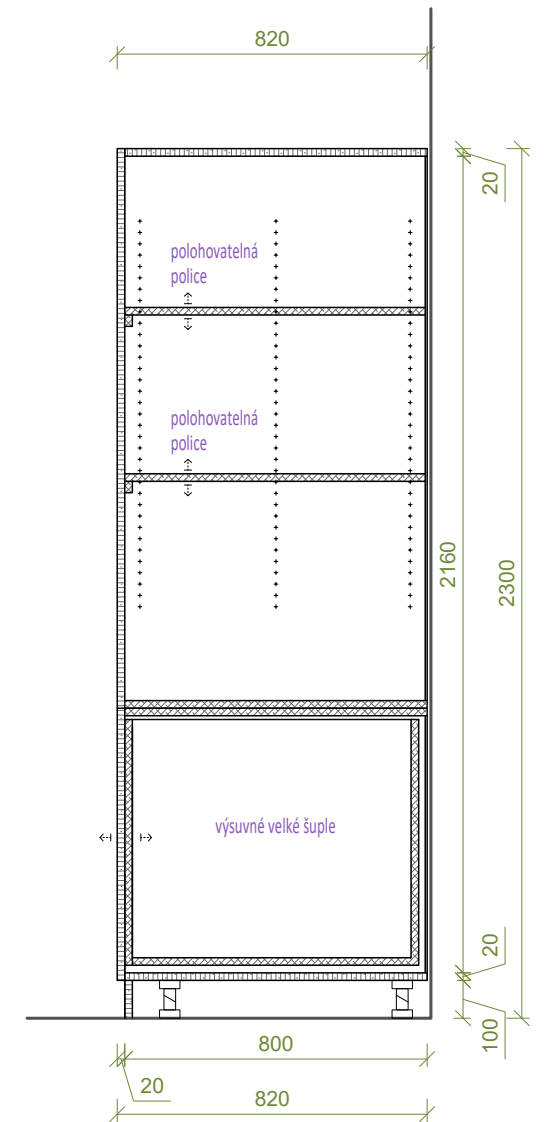
ŘEZ B-B
