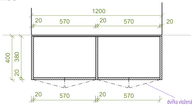
PŮDORYS 2
