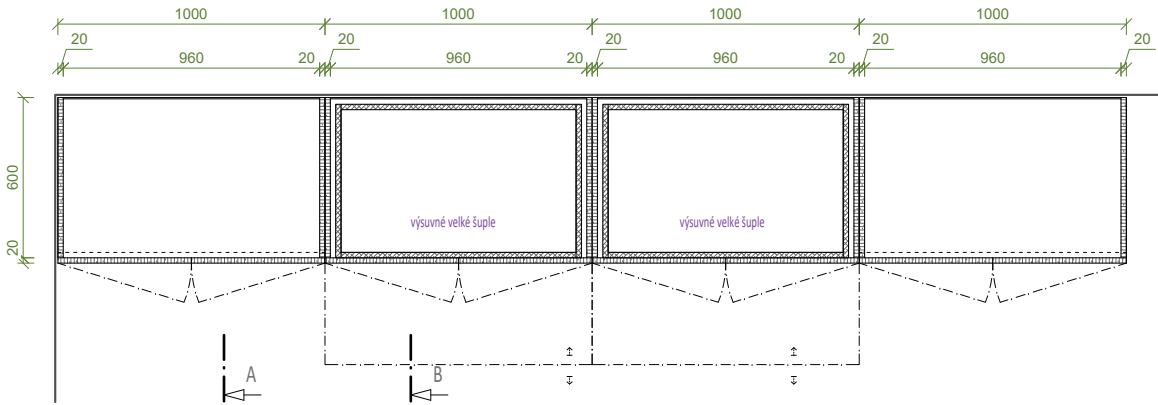
PŮDORYS
