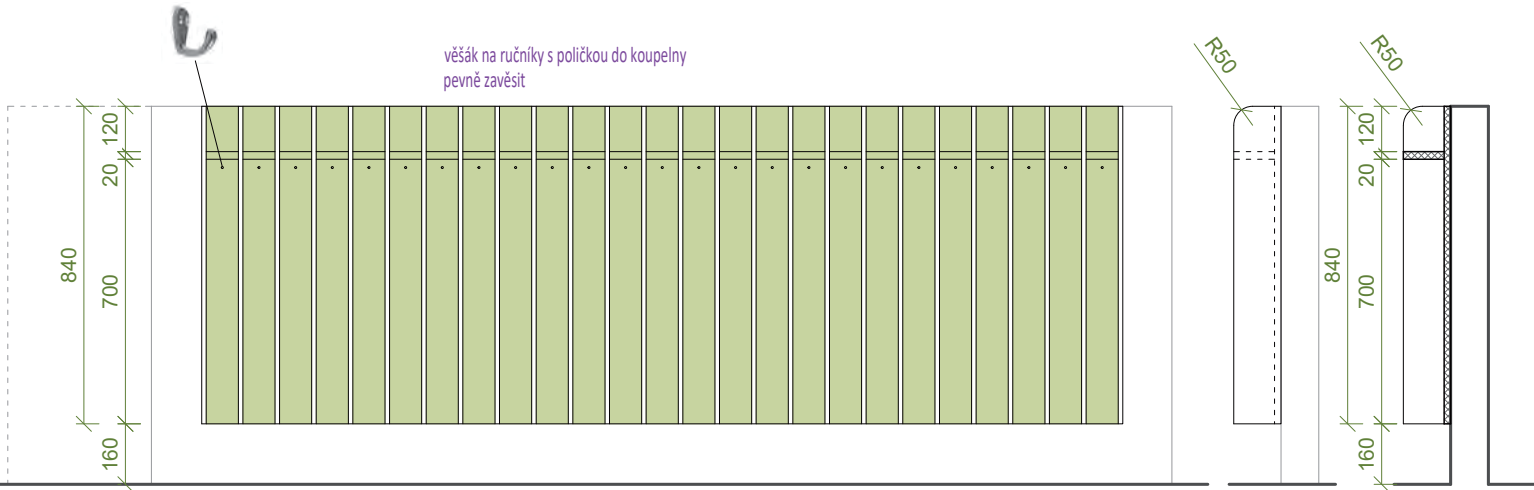
PŮDORYS
