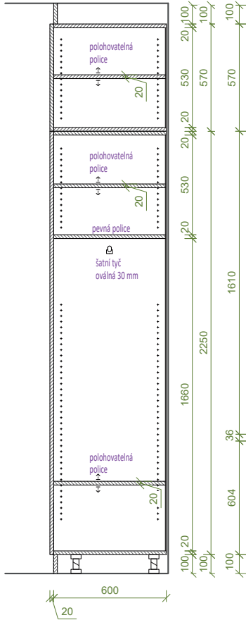
ŘEZ A-A
