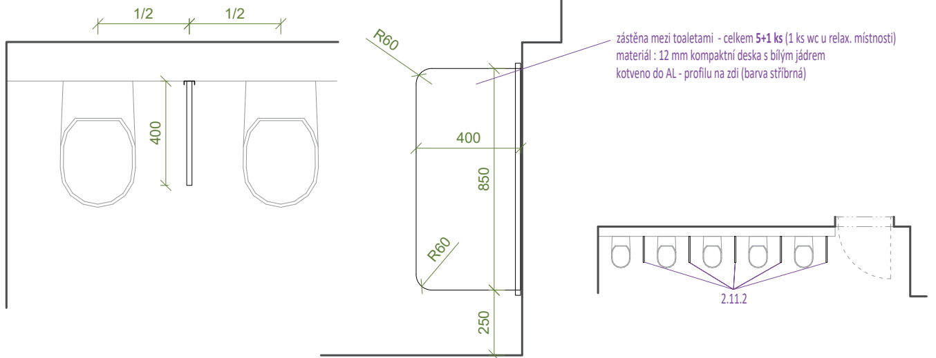
PŮDORYS
