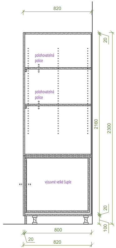
ŘEZ B-B
