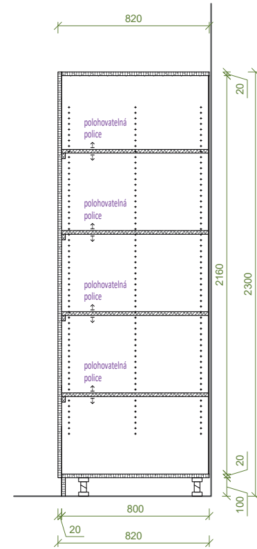
ŘEZ A-A
