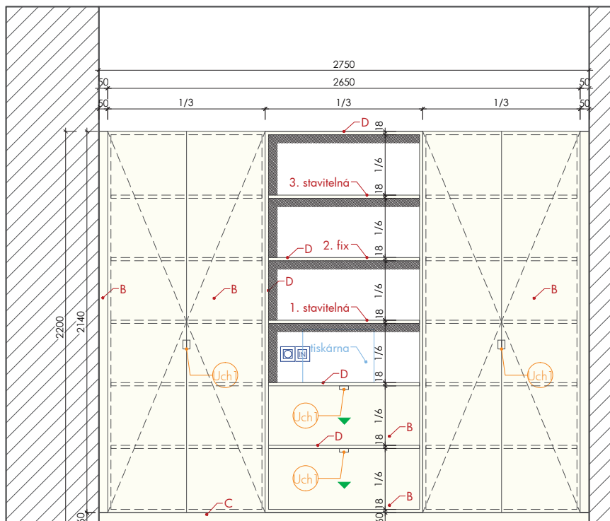
Čelní pohled
