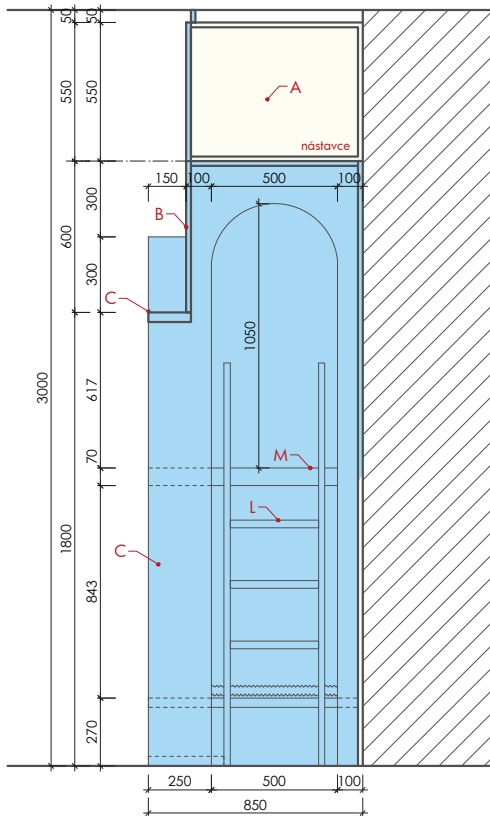
Řez BB'
