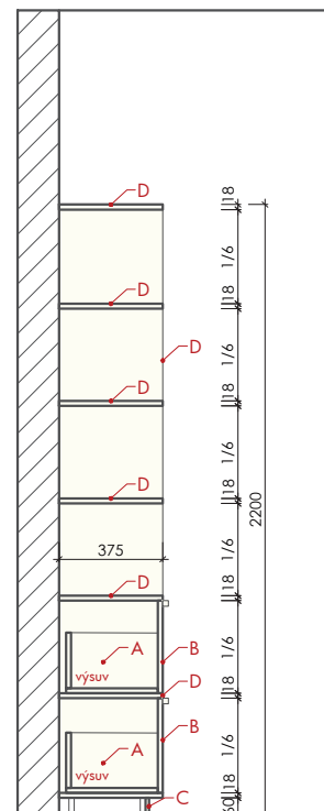
Řez AA'
