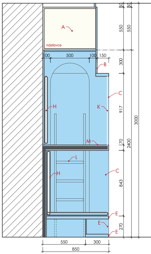
Řez AA'
